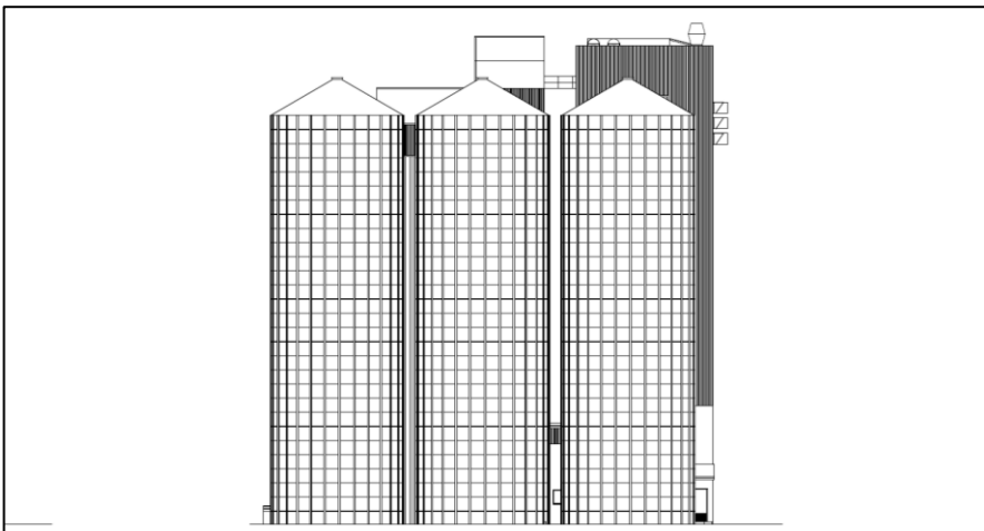
Fasadetegning i retning Dampsaga med inntegnet nye siloer på nordre side av dagens bygning.
